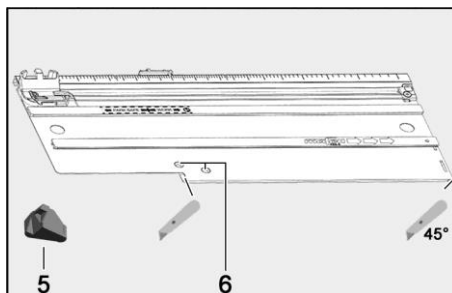
Fig. 44: Cortar la protección contra virutas
