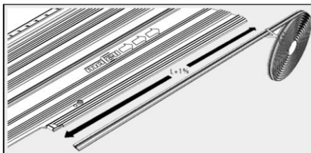
III. 29 : insertion du nouveau pare-éclats
