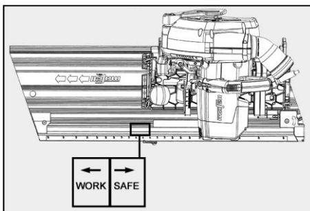
III. 23 : utilisation de la machine avec le dispositif de guidage
