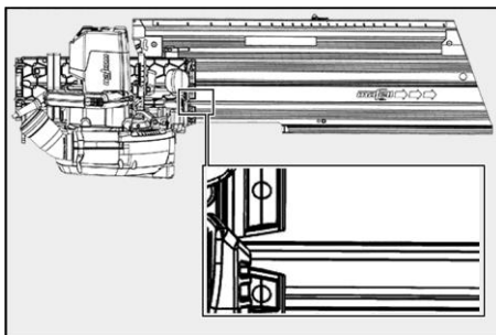
Fig. 38: Ajustar el ángulo de trabajo en el dispositivo guía
